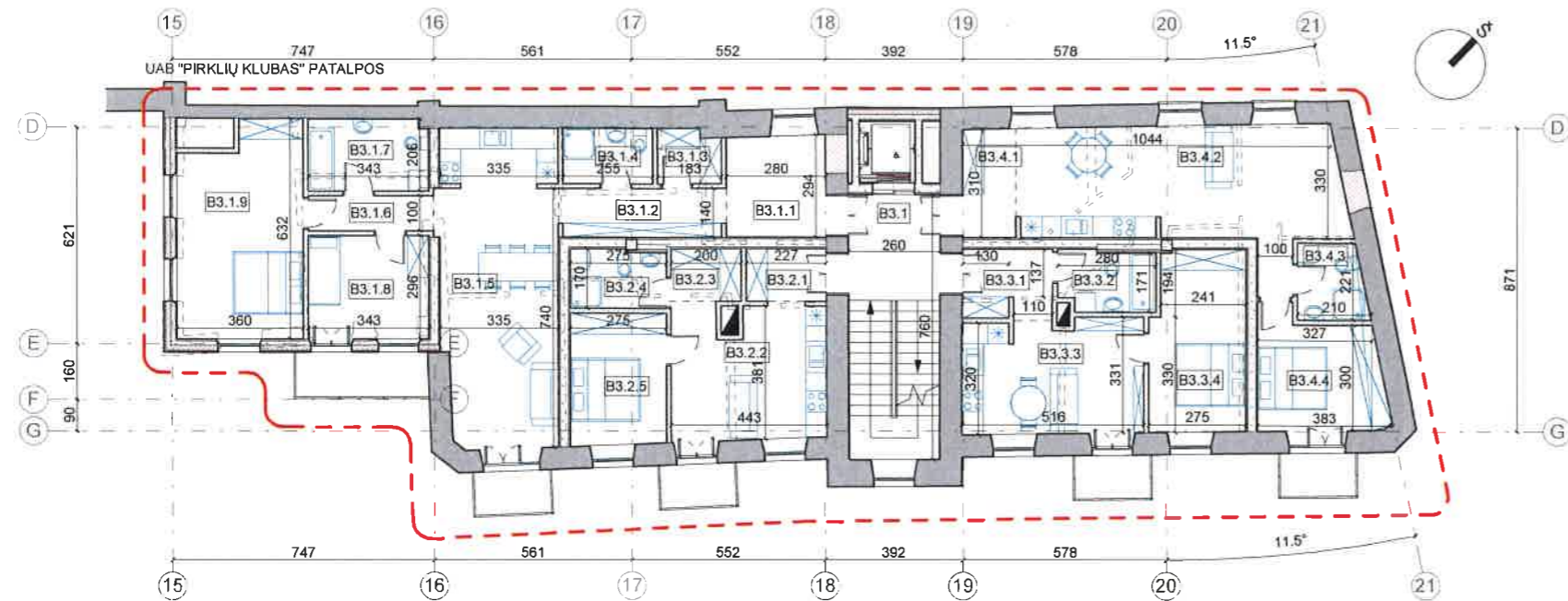
03-TREČIAS AUKŠTAS 1 : 200
