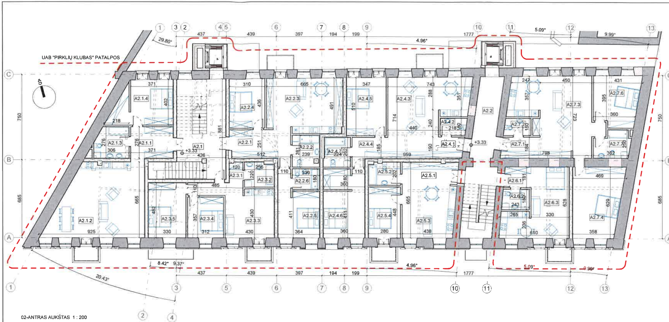
02-ANTRAS AUKŠTAS 1 : 200
