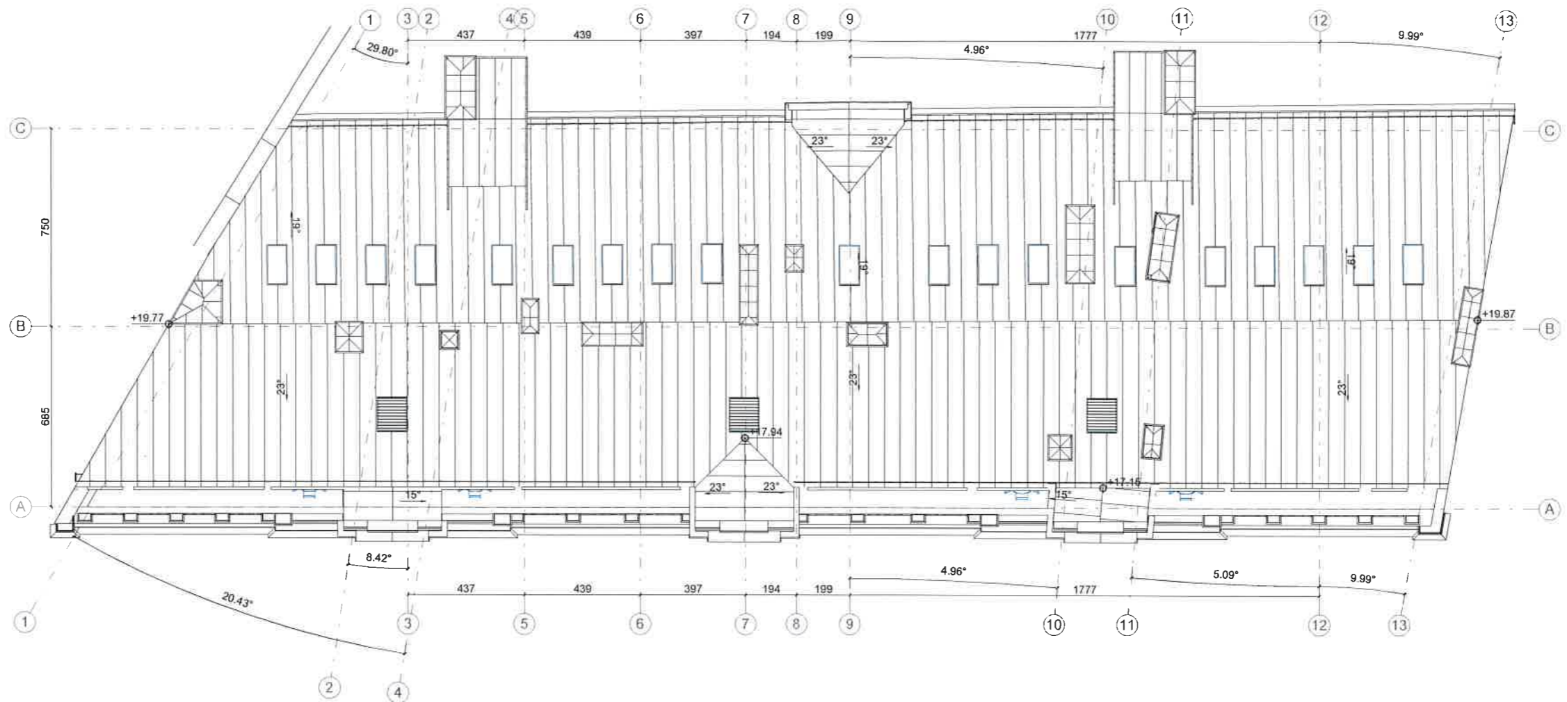
07-STOGAS 1 : 200
