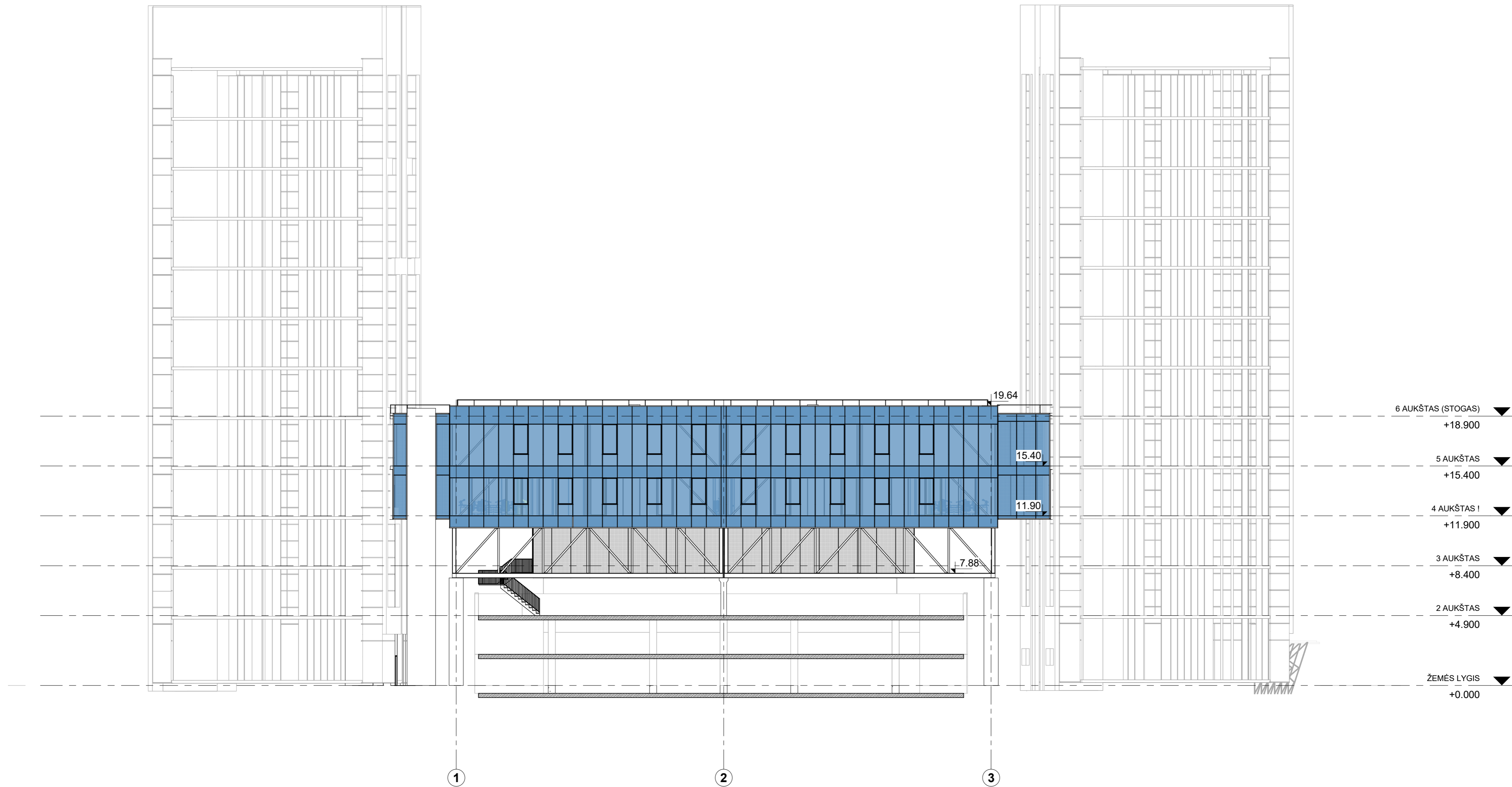
1 3 RYTINIS FASADAS 1 : 200
