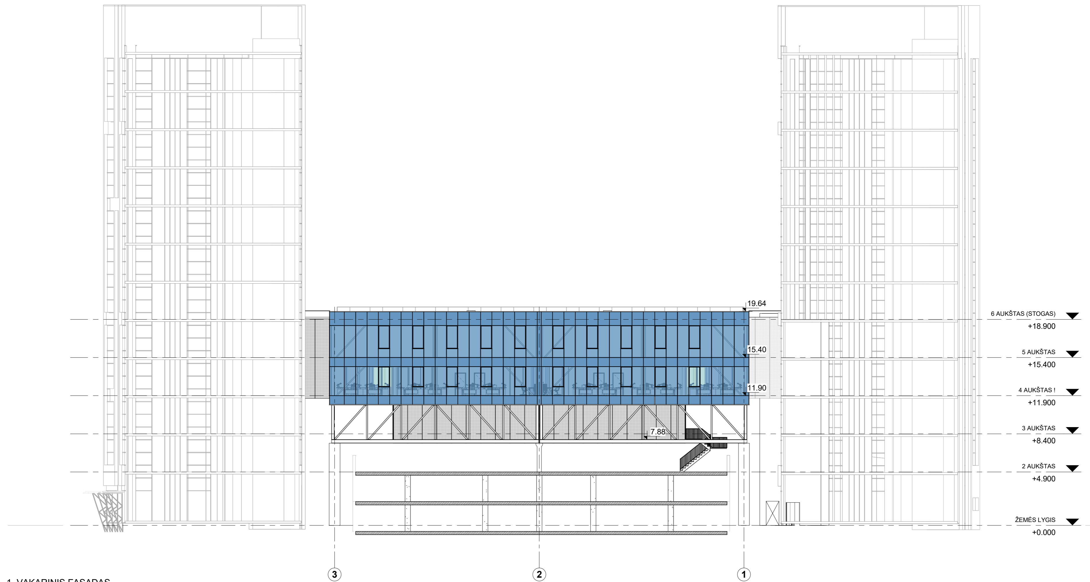
1. VAKARINIS FASADAS 1 : 200
